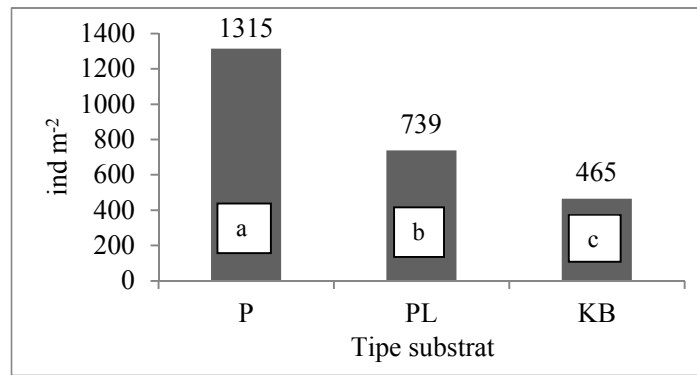
Gambar 5. Uji Kruskal-Wallis dan Uji Dunn perbandingan kelimpahan (ind/m 2 ) antar tipe substrat (P; Pasir, PL; Pasir+lumpur; KB; Kerikil-Batu) dari sembilan stasiun dan 12 bulan pengambilan contoh
