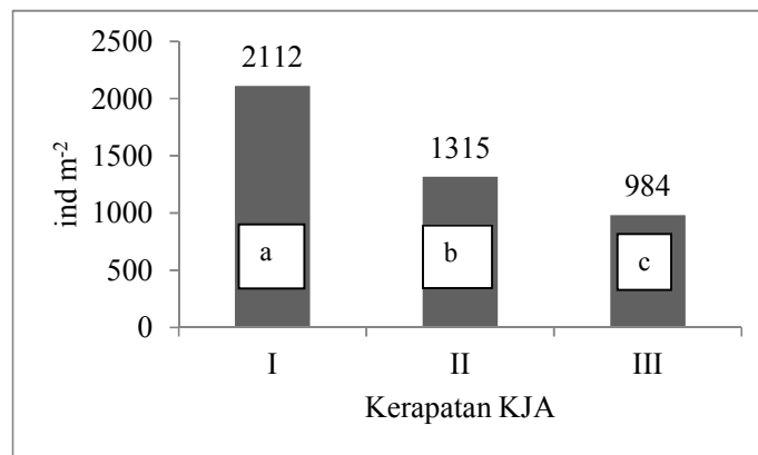
Gambar 6. Uji Kruskal-Wallis dan Uji Dunn perbandingan kelimpahan (ind/m 2 ) antar wilayah kerapatan KJA (I < 225 petak km -1 ; II 225 >< 675 petak km -1 ; III > 675 petak km -1 ) dari sembilan stasiun dan 12 bulan
